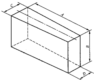
图 4 竖厚楔形砖
