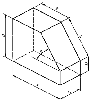
图 6 拱脚砖
